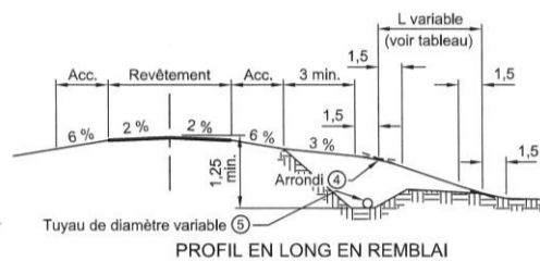
PROFIL EN LONG EN REMBLAI
